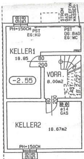
VOLLKELLER
