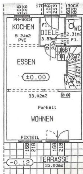
ERDGESCHOSS
