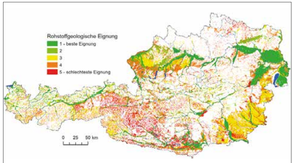
Abbildung 1: Rohstoffgeologische Eignung von Kiessandvorkommen in Österreich, aus Rohstoffplan2012, Rohstoffplan, bmlrt.gv.at
