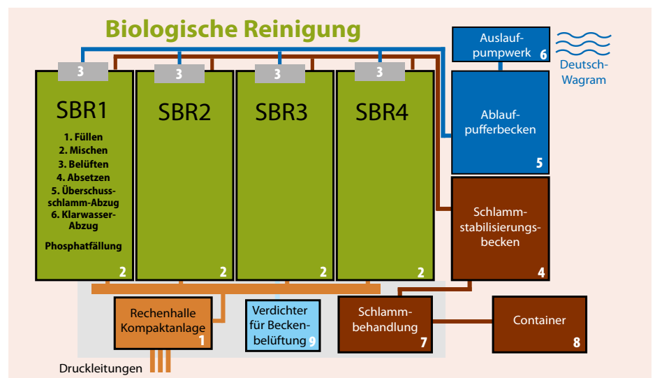
SBR (Sequencing Batch Reactor) Verfahren : Skizze des Aufbaus der Kläranlage (Grafik: GGK)
